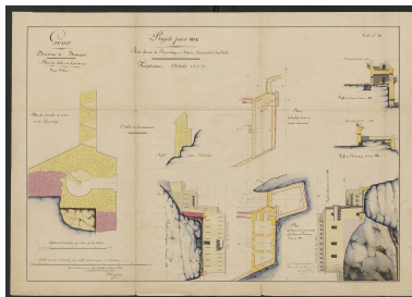
Place de Salins et dépendances. Bas-Belin. Projets pour 1838. Plate forme de l'hermitage et réduit casematé du bas Belin - Fortifications articles 15 et 17 (1838). IVR43_20223901204NUC4A
