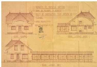
Projet de construction d'un atelier de mécanique [élévation des façades], 1935. IVR43_20192500043NUC4A
