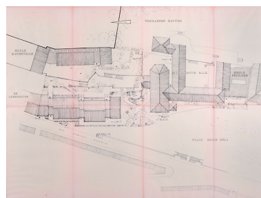
Ancien lycée Considerant. Plan d'aménagement, s.d. [1977]. Phot. Jérôme Mongreville IVR43_20233900919NUC4A
