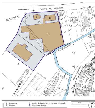
Plan-masse et de situation. Extrait du plan cadastral, 1984, section AI, 1:1000. Dess. André Céréza IVR43_20039000025NUDA
