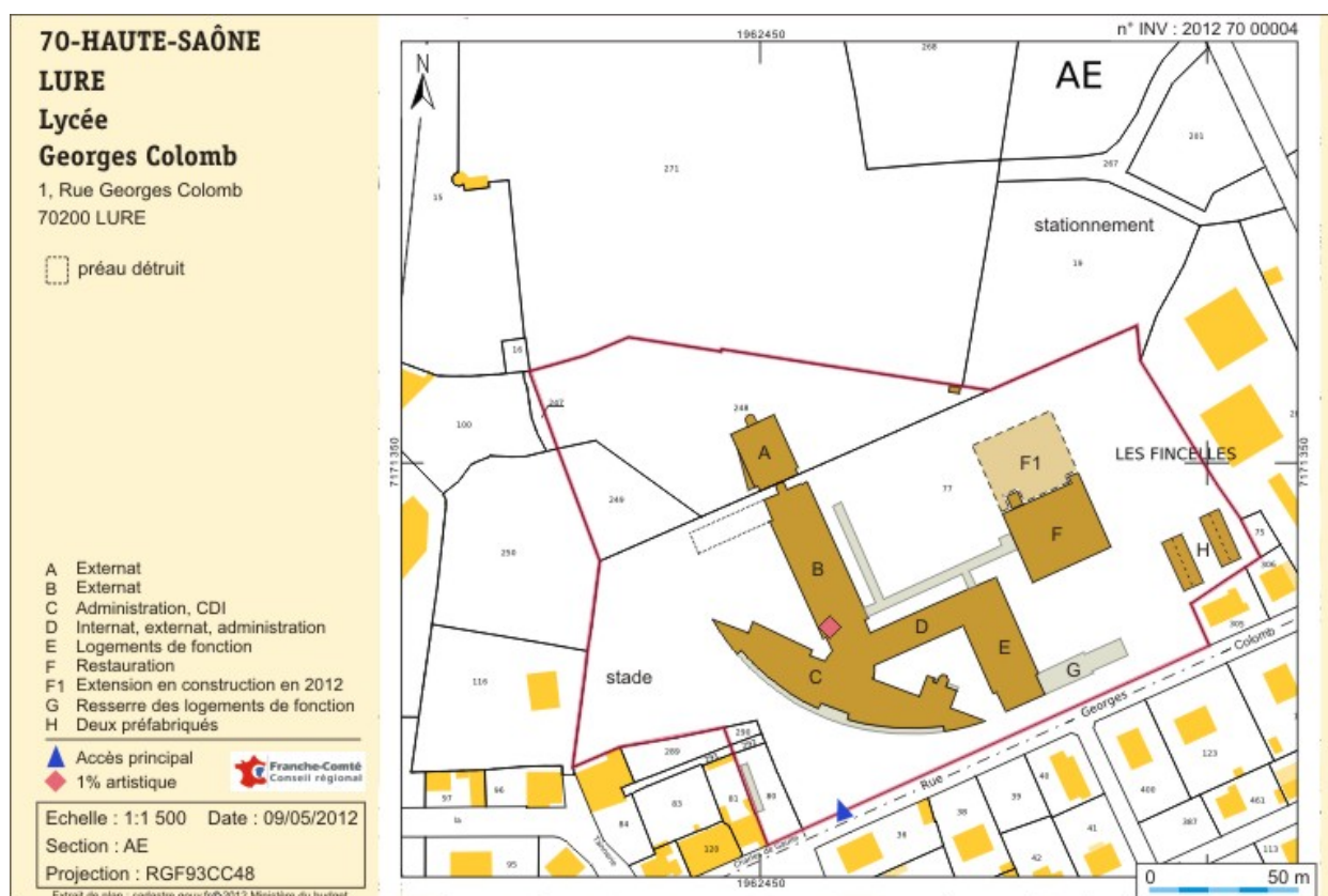
Plan-masse et de situation. Extrait du plan cadastral numérisé, sections AE, échelle 1:1500
