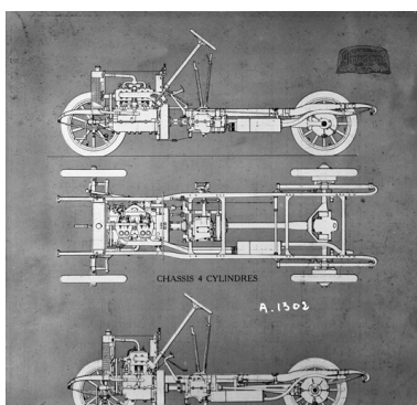
Plan d'un châssis équipé d'un moteur 4 cylindres. IVR43_20122501550NUC2
