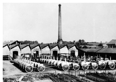
Département Chauffage. Fabrication des cuisines roulantes pendant la Première Guerre mondiale.
