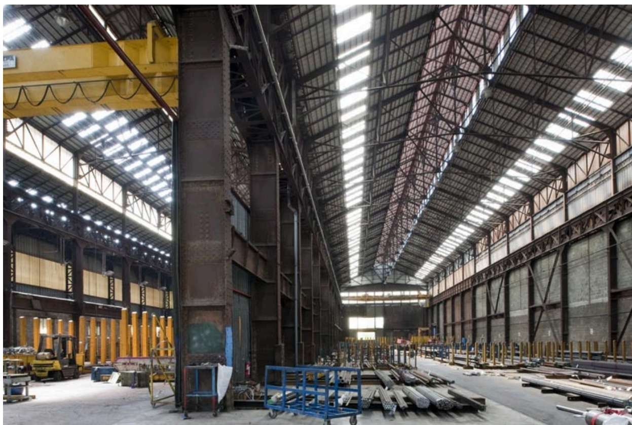
Halles de l'aciérie. Vue intérieure.
