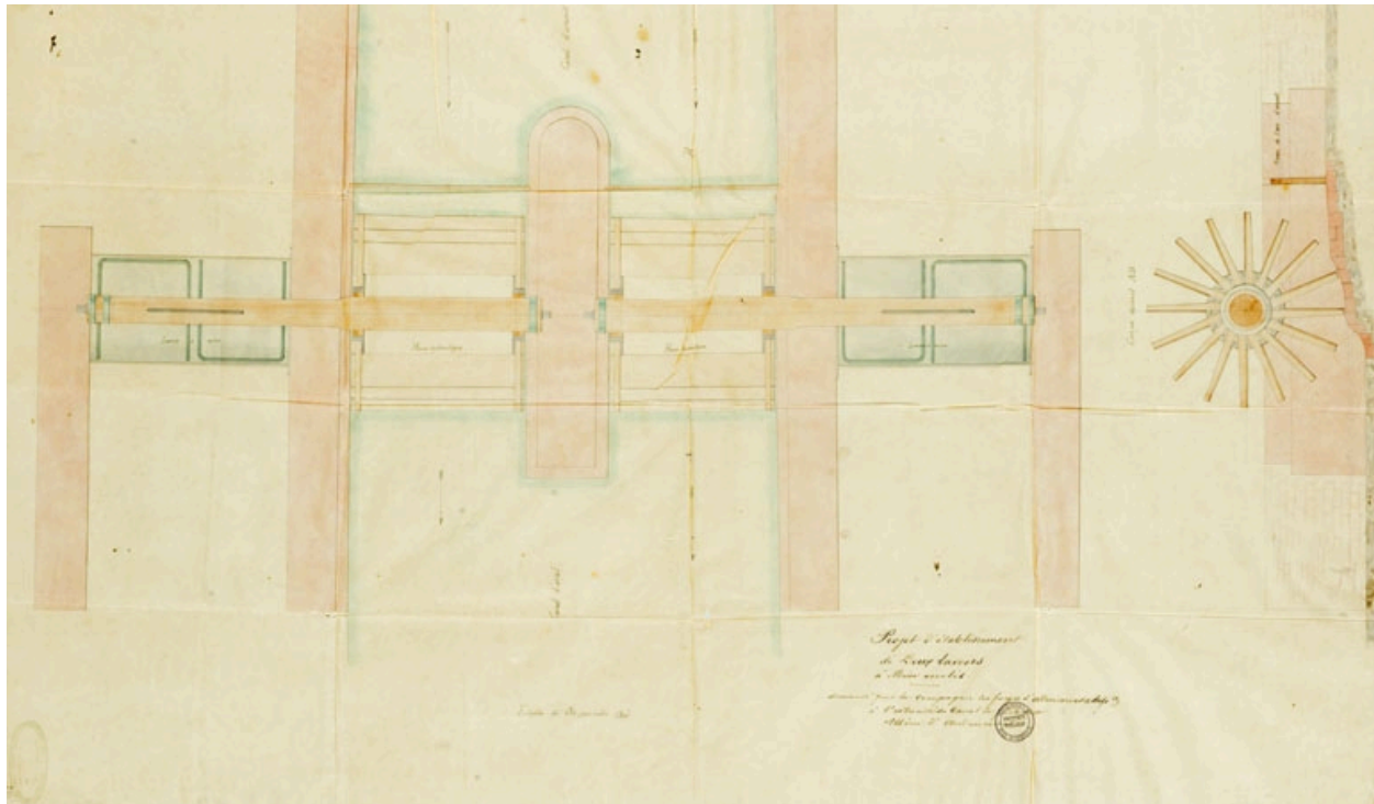
Projet d'établissement de deux lavoirs à mine accolés. Plan, s.n., s.d. [vers 1860], échelle 1/100.
