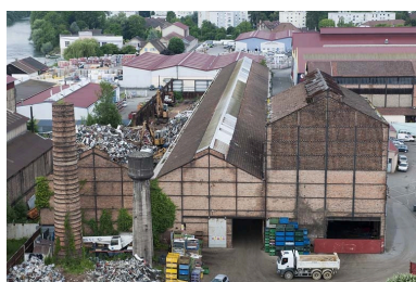
Vue plongeante sur l'atelier de laminage.
