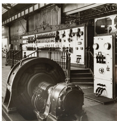
Alternateur et tableau électrique. Photogr., s.n., s.d. [milieu 20e siècle]. Phot. Jérôme Mongreville IVR43_20112500300NUC4A
