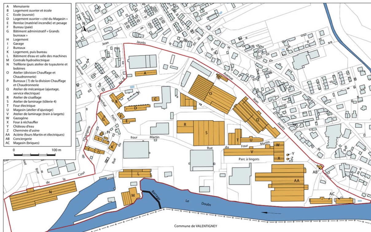
Plan-masse et de situation.
