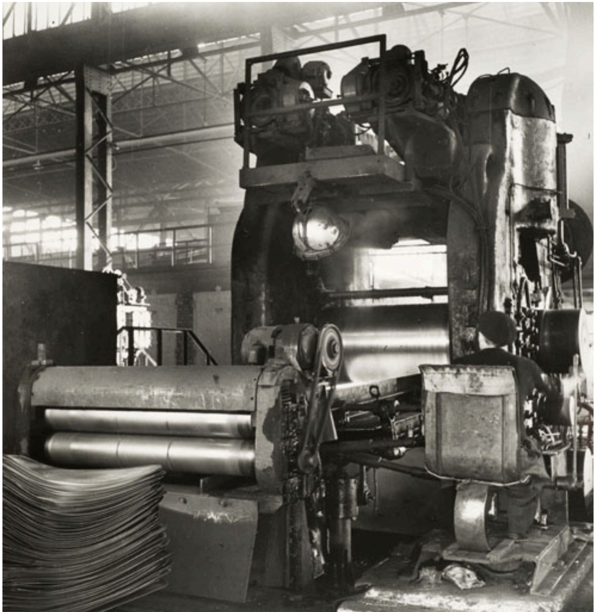
Le laminage des tôles. Photogr., s.n., s.d. [milieu 20e siècle].
