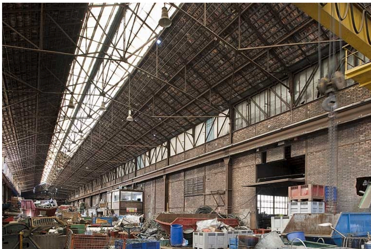
Atelier de laminage. Vue intérieure : charpente métallique et mur nord.
