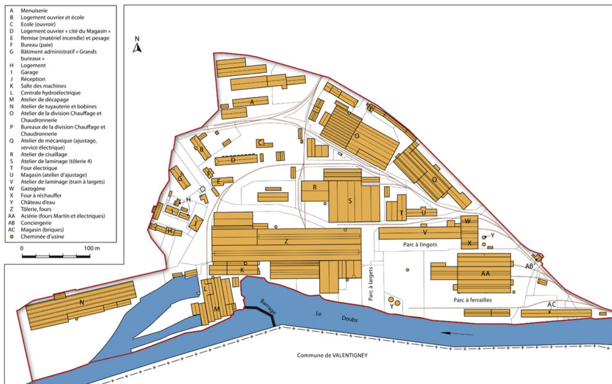
Plan-masse de l'usine vers 1970.
