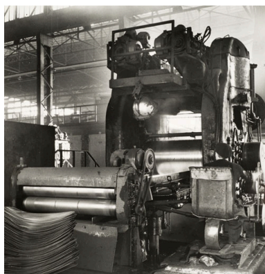
Le laminage des tôles. Photogr., s.n., s.d. [milieu 20e siècle]. Phot. Jérôme Mongreville IVR43_20112500299NUC4A
