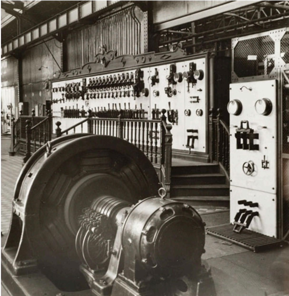
Alternateur et tableau électrique. Photogr., s.n., s.d. [milieu 20e siècle].
