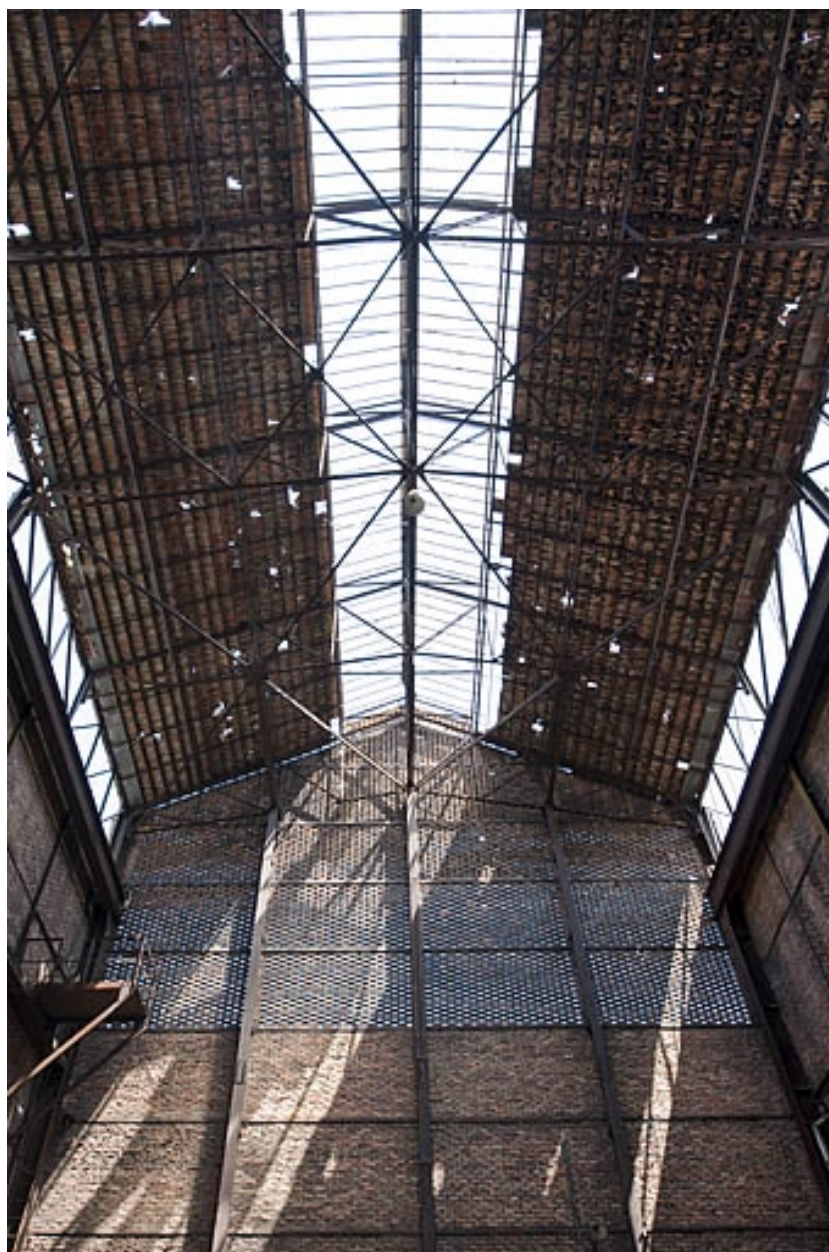
Vue intérieure du bâtiment du gazogène. Pignon est et charpente métallique.
