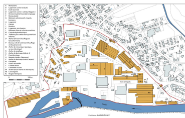
Plan-masse et de situation. Dess. Mathias Papigny IVR43_20132502534NUDA
