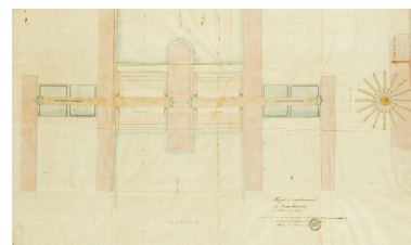
Projet d'établissement de deux lavoirs à mine accolés. Plan, s.n., s.d. [vers 1860], échelle 1/100. Phot. Jérôme Mongreville IVR43_20112500314NUC4A
