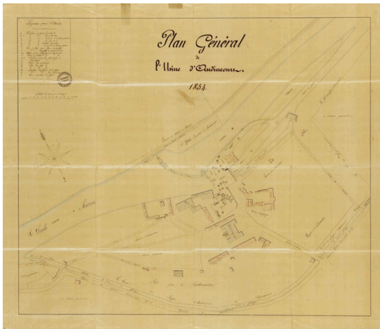
Plan général de l'usine d'Audincourt. Plan (plume, lavis, toile), 1854, s.n., échelle 1/1250.
