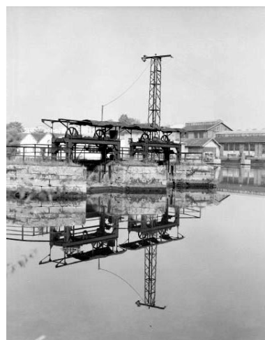
Vannage du barrage en 1981. Phot. Yves Sancey IVR43_19812500340X
