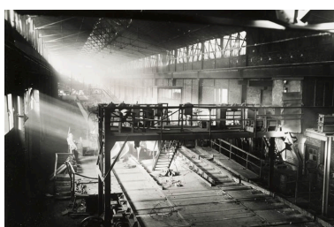
Halle de fonderie. Photogr., s.n., s.d. [milieu 20e siècle]. Phot. Jérôme Mongreville IVR43_20112500288NUC4A
