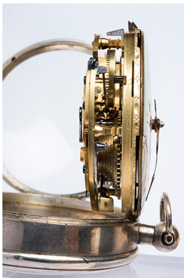
Vue de profil du mouvement. La fusée est visible dans la moitié inférieure. Phot. Sonia Dourlot IVR43_20182501627NUC4A
