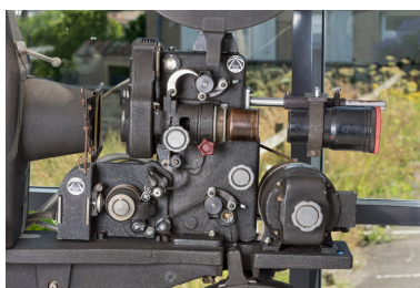
1er projecteur : chrono (bloc de projection, avec optique et moteur électrique). Phot. Pierre-Marie Barbe-Richaud IVR26_20257100697NUC4A
