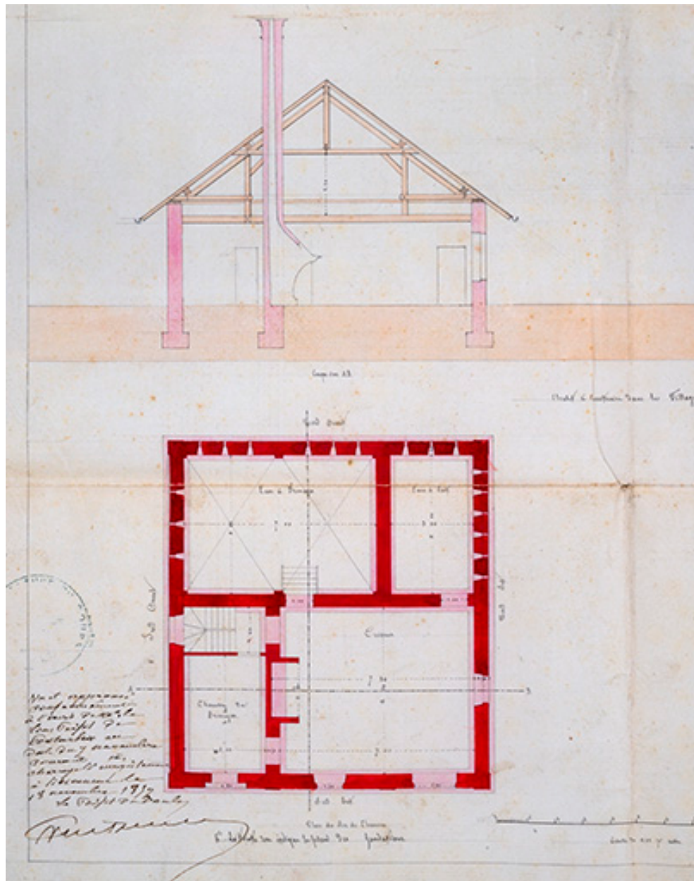
Projet de construction de trois chalets communaux [plan du rez-de-chaussée et coupe transversale], 1859.
