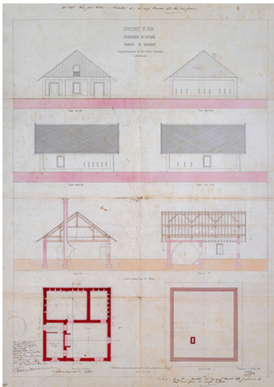
Projet de construction de trois chalets communaux, 1859.
