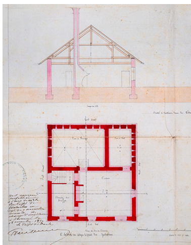
Projet de construction de trois chalets communaux [plan du rez-de- chaussée et coupe transversale], 1859. IVR43_20192500053NUC4A
