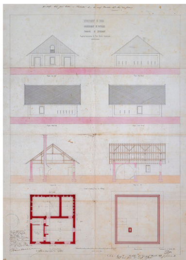
Projet de construction de trois chalets communaux, 1859. IVR43_20192500052NUC4A
