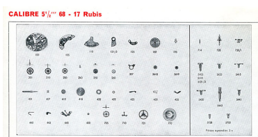
Calibre 5 1/2''' 68 - 17 rubis [éclaté des fournitures], 1973.
