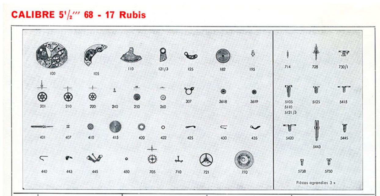
Calibre 5 1/2''' 68 - 17 rubis [éclaté des fournitures], 1973.
