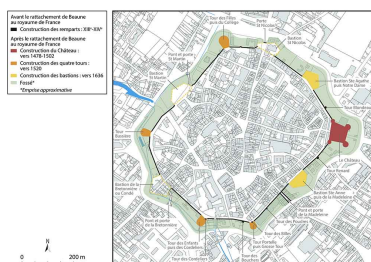
Plan de situation des fortifications de Beaune, 1/4 000.
