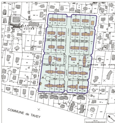
Plan-masse et de situation. Extrait du plan cadastral numérisé, 2005, section AS, 1:1000 réduit à 1:2000. Dess. André Céréza IVR43_20067000035NUDA
