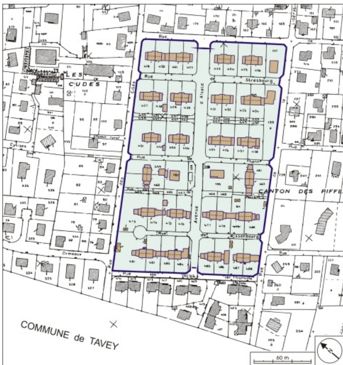
Plan-masse et de situation. Extrait du plan cadastral numérisé, 2005, section AS, 1:1000 réduit à 1:2000.
