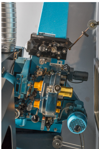
Chrono, tourelle porte-objectifs et module son. Phot. Pierre-Marie Barbe-Richaud IVR26_20257100187NUC4A
