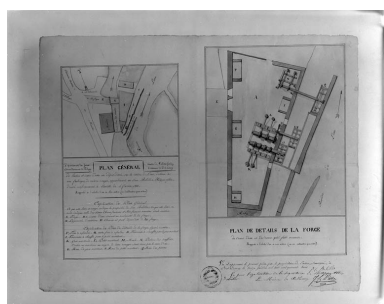
Plan général de l'usine [...] et plan de détails de la forge [...]. Phot. Jérôme Mongreville IVR43_19963901787V
