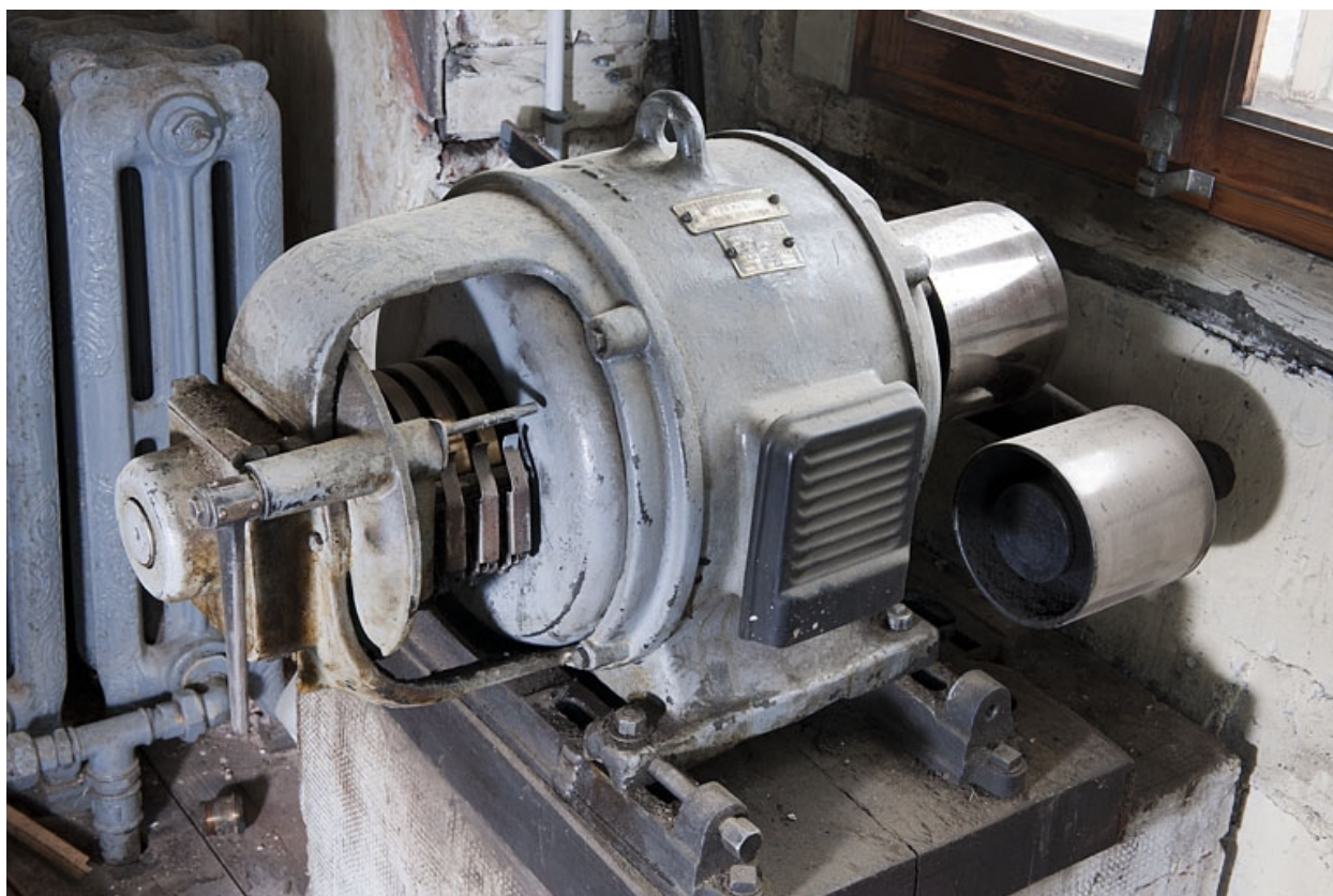
Moteur électrique.
