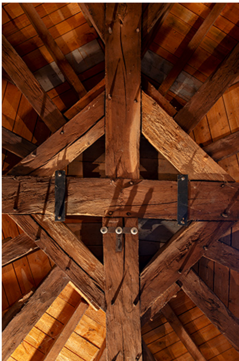
Charpente du dôme. Enrayure centrale.
