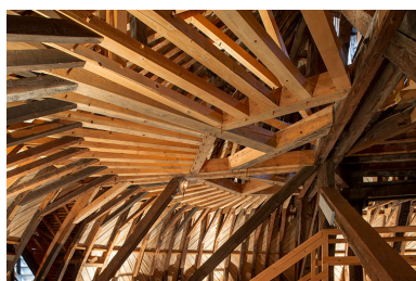
Enrayure du côté occidentale, depuis le sud. Phot. Nicolas Waltefaugle IVR43_20253900349NUC4A
