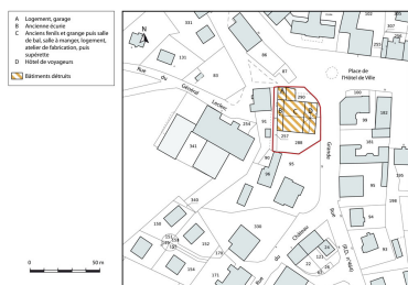
Plan-masse et de situation. Extrait du plan cadastral, 2015, section AI. Dess. Mathias Papigny IVR43_20152500671NUDA
