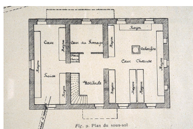
Plan du sous-sol.
