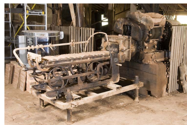
Mouleuse-étireuse Brandt et broyeur Dubois. Phot. Jérôme Mongreville IVR43_20087000780NUC2A
