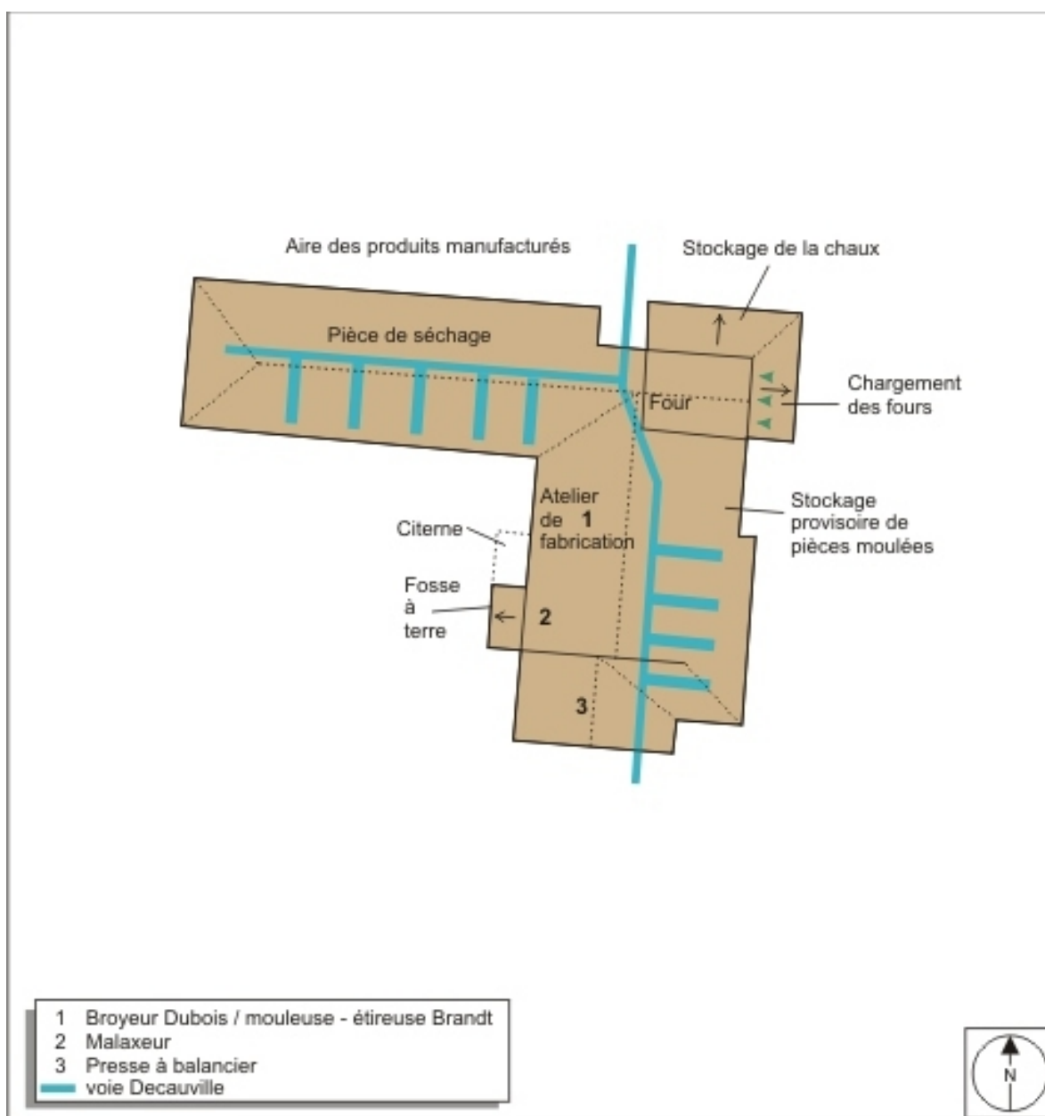
Plan-masse des bâtiments de production. Mis au net A. Céréza, d'après l'extrait du plan cadastral numérisé, 2008, section ZB.
