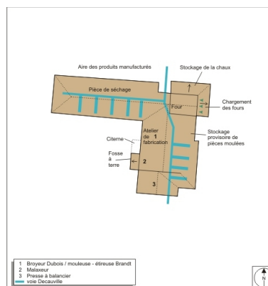
Plan-masse des bâtiments de production. Mis au net A. Céréza, d'après l'extrait du plan cadastral numérisé, 2008, section ZB. Dess. André Céréza IVR43_20087000993NUDA
