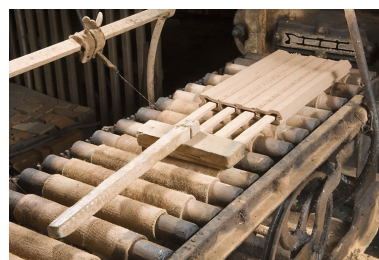
Chariot de découpe de la mouleuse-étireuse. Enlèvement d'une brique creuse. Phot. Jérôme Mongreville IVR43_20087000784NUC2A
