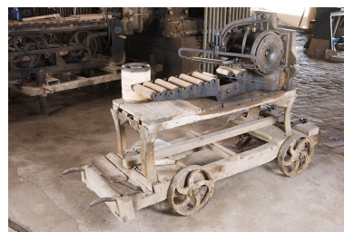
Mouleuse-étireuse pour tuiles sur son chariot découpeur. Phot. Jérôme Mongreville IVR43_20087000788NUC2A
