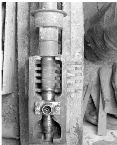
Clavier ouvert : filetage de l'arbre du tour et clés de sélection. Filetage standard à gauche, filetage fin à droite. Phot. Jérôme Mongreville IVR43_19943901203X
