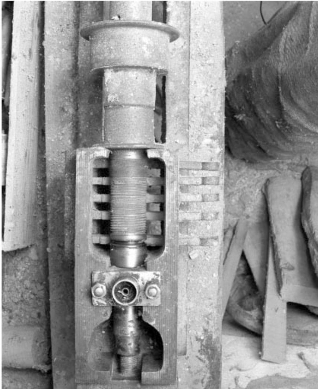
Clavier ouvert : filetage de l'arbre du tour et clés de sélection. Filetage standard à gauche, filetage fin à droite.
