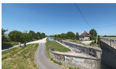
Site vu d'aval. Le désaxement du pont sur écluse par rapport au sas est nettement visible. Phot. Thierry Kuntz IVR26_20112103019NUC4A
