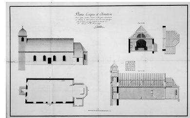
Plan, coupes et élévation d'une église [...], 1817. Phot. Jérôme Mongreville, Autr. Elmerich IVR43_19872500241X
