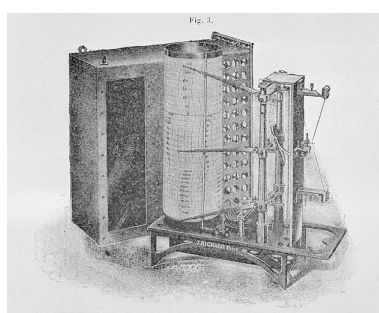
[Enregistreur baro-thermo-hygromètre Jules Richard utilisé lors de la mission d'observation de l'éclipse de soleil à Cistierna en 1905].
