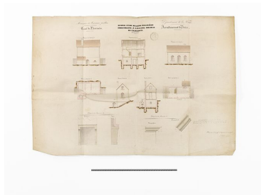
"Dessin d'une maison éclusière construite à l'écluse double de Chavance". Plan, coupe et élévation (avec détails de la cheminée et de la corniche). (Dessin ; 1854 ; 84 x 56,5 cm, Archives VNF-direction territoriale Centre-Bourgogne ; subdivision de Corbigny) Phot. Thierry Kuntz IVR26_20135800023NUC4A
