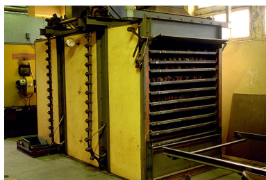
Vue d'ensemble de trois quarts droit. Séchoir ouvert avec ses 10 grilles. Phot. Jérôme Mongreville IVR43_19973900707ZA
