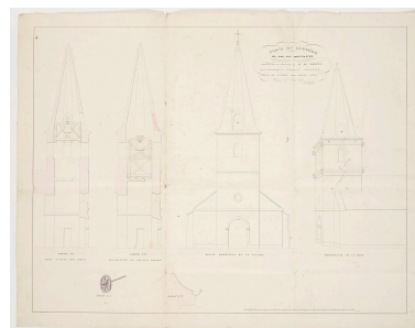
Plans du clocher de Fay-en-Montagne. Coupe n°1. Coupe n°2. Dessin géométral de la façade. Perspective de la tour. 1839. Autr. Perrard IVR43_20243901228NUC4A
