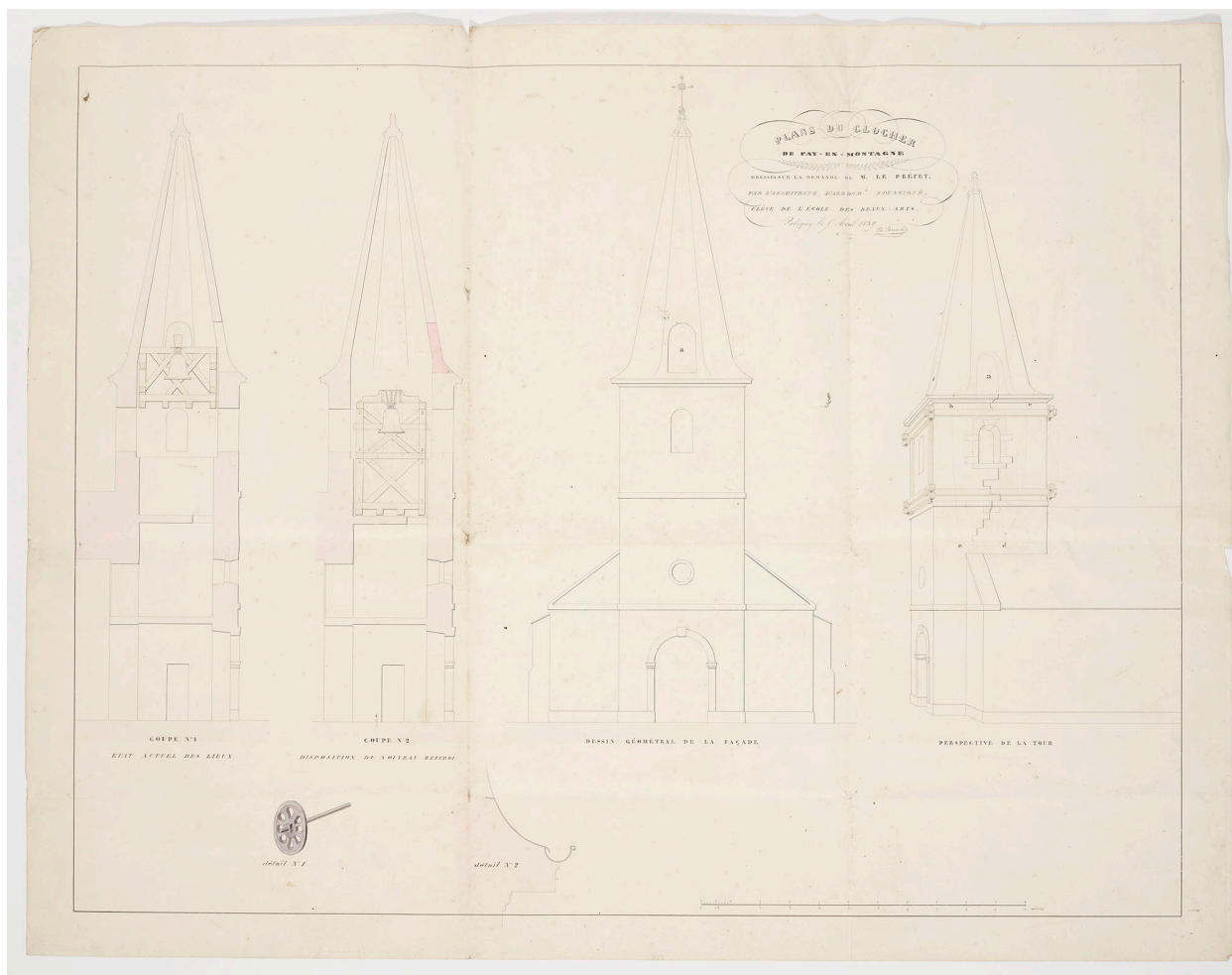
Plans du clocher de Fay-en-Montagne. Coupe n°1. Coupe n°2. Dessin géométral de la façade. Perspective de la tour. 1839.
