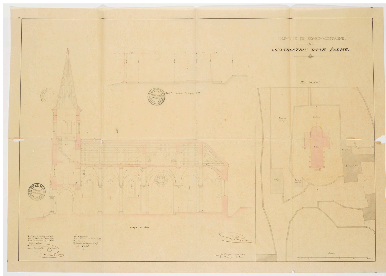
Construction d'une église. Plan général. Coupe en long. Profil. 1855.
