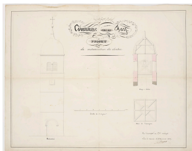
Projet de restauration du clocher. Elévation. Coupe du clocher. Plan de l'enrayure. 1838. Autr. René Léon Victor Pourchot IVR43_20243901231NUC4A
