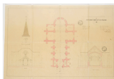
Construction d'une église. Elévation. Plan. Coupe en travers. 1855. Autr. Achille Paillot IVR43_20243901233NUC4A
