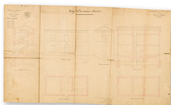
Projet de la maison éclusière. Travaux du Châtelet. Plans, coupes et élévations. Phot. Thierry Kuntz, Autr. François Anus IVR26_20197100704NUC4A
