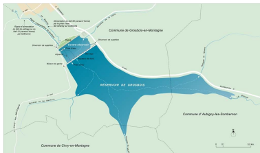
Plan schématique d'ensemble du réservoir de Grosbois.
