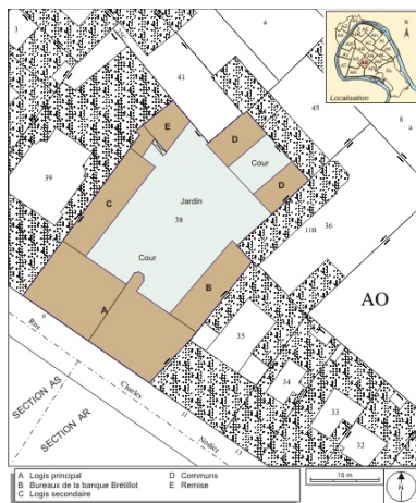
Plan masse et de situation. Extrait du plan cadastral, 1993, section AO. Dess. André Céréza IVR43_20072500017NUDA
