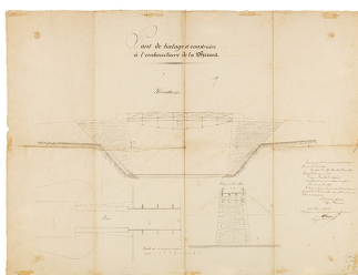
Pont de halage à construire à l'embouchure de la Dheune. Plan, coupe et élévation. Dessin, 30 août 1837. Phot. Thierry Kuntz IVR26_20217100009NUC4A
