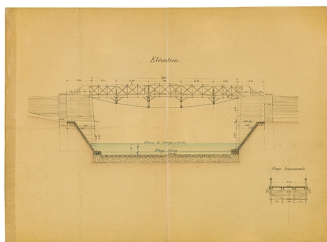
Reconstruction du pont de halage de la Dheune. Dessins du pont actuel. [Elévation et coupe transversale]. Dessin aquarellé, 24 janvier 1903.
