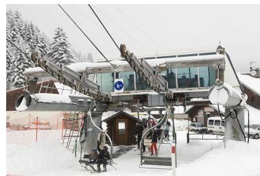
Arrivée aux Tavins du télésiège provenant du domaine de Piquemiette. Phot. Jérôme Mongreville IVR43_20092500163NUC2A
