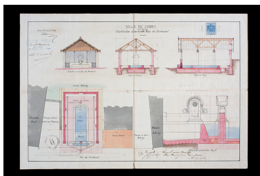
Plan, élévations, coupes et vue de détail de la fontaine-lavoir rue du Parlement à Jussey, 1869. Phot. Nicolas Waltefaugle IVR43_20257000212NUC4A
