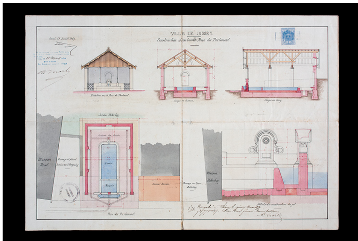
Plan, élévations, coupes et vue de détail de la fontaine-lavoir rue du Parlement à Jussey, 1869.
