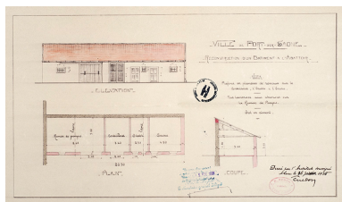
Reconstruction d'un bâtiment à l'abattoir : plan, coupe et élévation. Phot. Jérôme Mongreville, Autr. auteur inconnu IVR43_20177001160NUC4A
