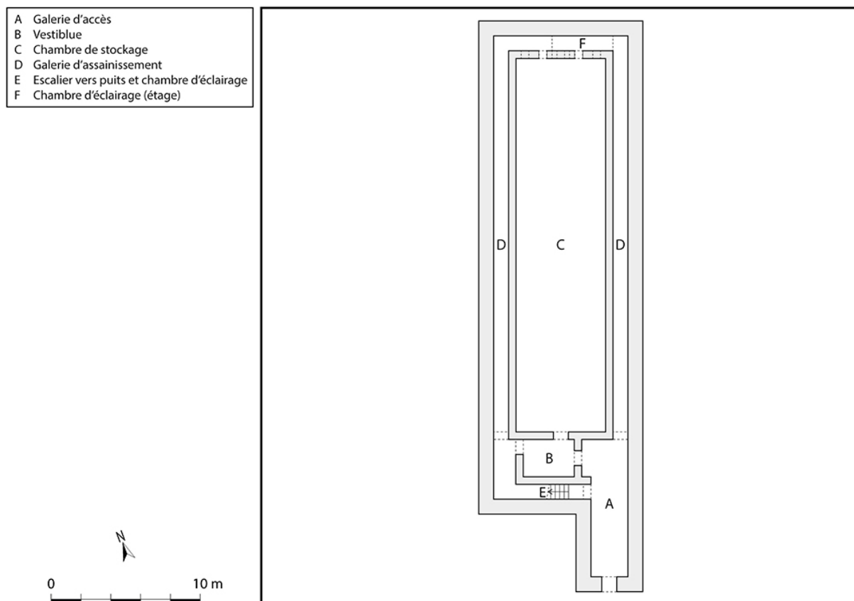
Plan masse et de situation. 1/200.
