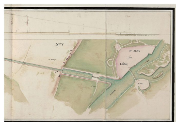
"Plans et nivellements pour un projet de canal de Dijon à Saint-Jean-de-Lône le long des coteaux.
