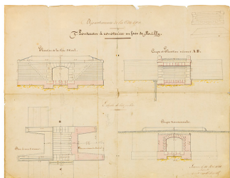
Ponceau à construire en face de Pouilly. Plan, coupe et élévation. Dessin, 30 mai 1844.
