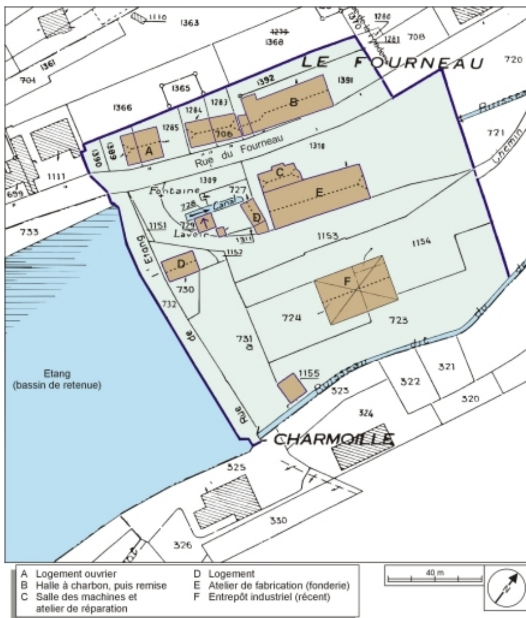
Plan-masse et de situation. Extrait du plan cadastral numérisé, 2005, section A, 1:1250.
