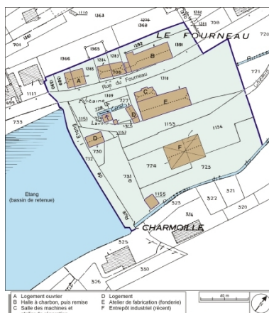
Plan-masse et de situation. Extrait du plan cadastral numérisé, 2005, section A, 1:1250. Dess. André Céréza IVR43_20067000067NUDA
