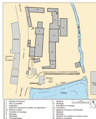
Plan-masse de la fonderie en 1930. Dess. André Céréza IVR43_20067000001NUDA
