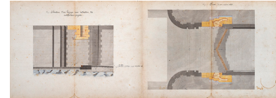
Construction du barrage mobile et de la seconde porte de garde de St-Albin - Porte de garde amont (1876). Phot. Jérôme Mongreville, Autr. Gustave Bouvaist IVR43_20207000067NUC4A
