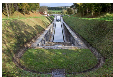
Vue amont du canal. Phot. Sonia Dourlot IVR43_20157000211NUC2A
