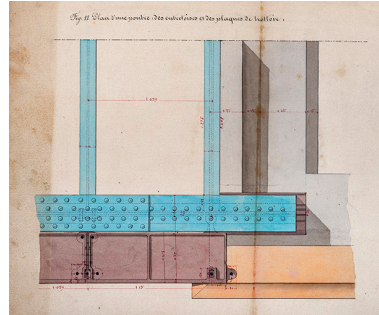
Réfection de la première porte de garde de la dérivation de St-Albin - Plans, élévation, coupes et détails des maçonneries de la porte de garde et du pont (1876) : plan d'une poutre, des entretoises et des plaques de trottoirs. Phot. Jérôme Mongreville, Autr. Gustave Bouvaist IVR43_20207000066NUC4A
