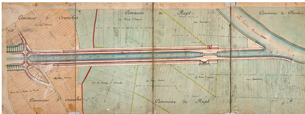
Achèvement de la dérivation de St-Albin (en aval du souterrain) - Plan général (1876).
