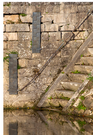
Echelles limnimétriques, porte de garde. Phot. Sonia Dourlot IVR43_20157000217NUC2A
