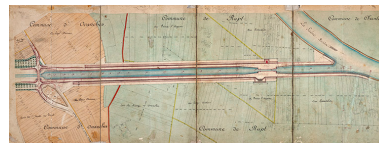
Achèvement de la dérivation de St-Albin (en aval du souterrain) - Plan général (1876). Phot. Jérôme Mongreville, Autr. Gustave Bouvaist IVR43_20207000075NUC4A
