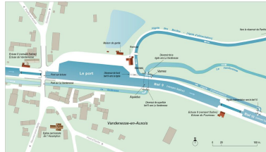
Plan schématique du port et du réseau hydraulique. Dess. Alain Morelière IVR26_20132100099NUDA
