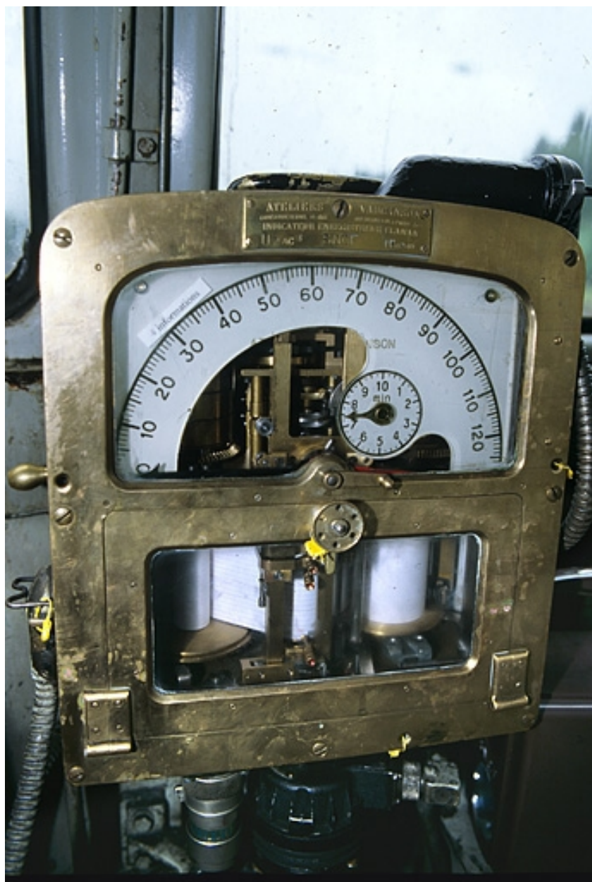
Intérieur, côté extrémité 1 : indicateur - enregistreur Flaman.
