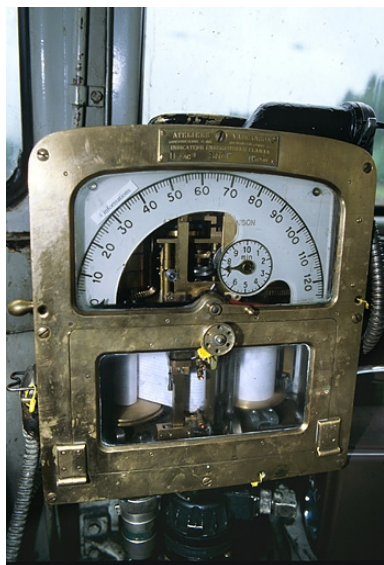
Intérieur, côté extrémité 1 : indicateur - enregistreur Flaman. Phot. Yves Sancey IVR43_20053900020ZA
