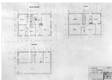
Vouglans. Cité d'exploitation. Maison n° 2 vue en plan. Phot. Jérôme Mongreville, Autr. B.V. IVR43_19913900723V
