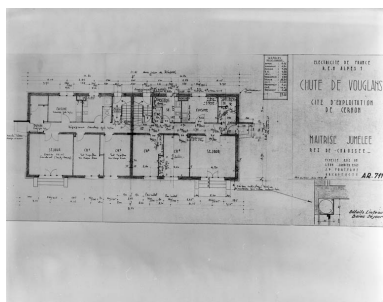
Electricité de France [...] Cité d'exploitation de Cernon. Maîtrise jumelée. Rez-de-chaussée. Phot. Jérôme Mongreville, Autr. J.-P. Fonterne IVR43_19913900722V
