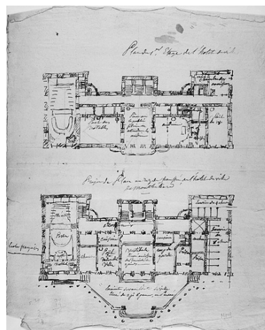
Projet de plan au rez-de- chaussée [...] et Plan du 1er étage [...], vers 1771-1772. Phot. Jérôme Mongreville, Autr. Pierre-Louis- Philippe de (?) La Guépière IVR43_19872500085V
