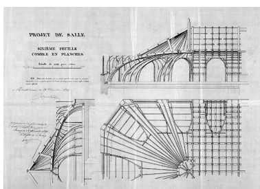
Projet de salle de spectacle (...] Combles en planches, 1854. Phot. Jérôme Mongreville, Phot. Auguste Goguel IVR43_19872500218X
