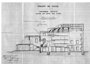
Projet de salle de spectacle (...] Coupe en long sur l'axe, 1854. Phot. Jérôme Mongreville, Phot. Auguste Goguel IVR43_19872500217X
