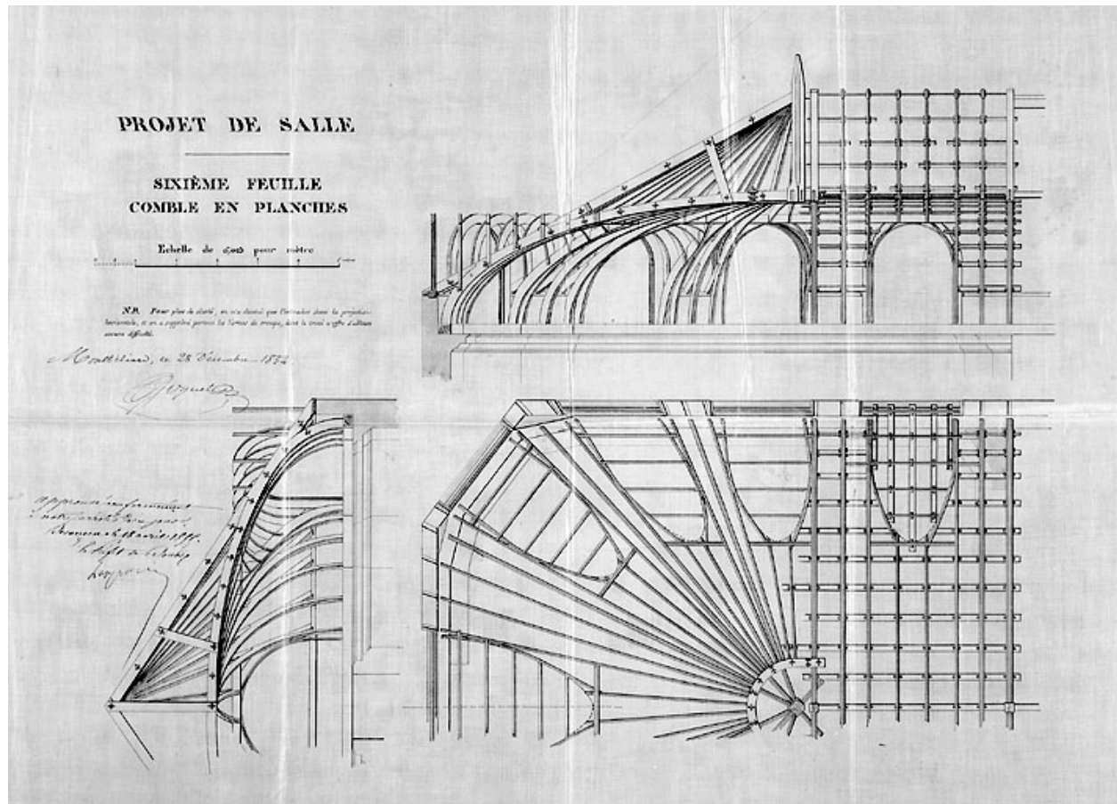
Projet de salle de spectacle [...] Combles en planches, 1854.
