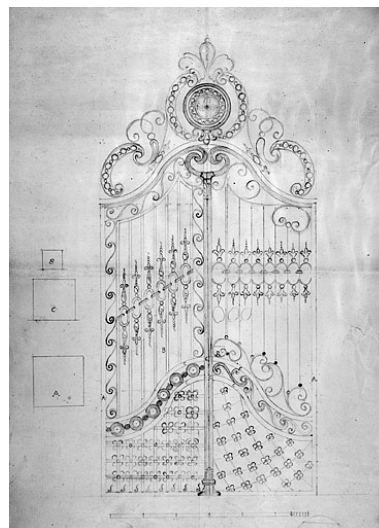
Projet de grille [pour les cours], vers 1776-1777. Phot. Jérôme Mongreville IVR43_19872500091V
