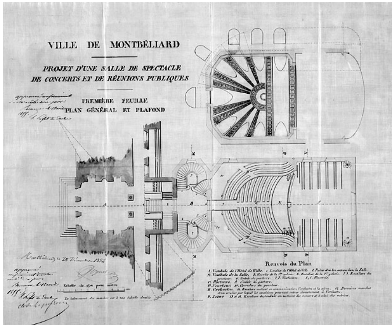
Projet de salle de spectacle (...) Plan général et plafond, 1854.
