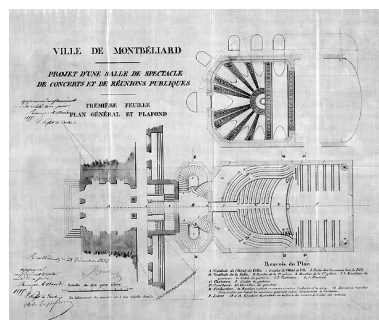
Projet de salle de spectacle (...] Plan général et plafond, 1854. Phot. Jérôme Mongreville, Phot. Auguste Goguel IVR43_19872500216X
