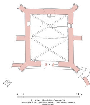
Plan de la chapelle. Dess. Alain Morelière IVR26_20132100067NUDA
