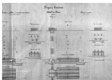
Usine de Fraisans. Détail des fours [les fours à souder].
