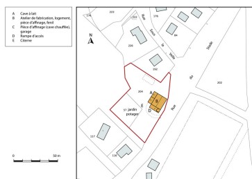
Plan-masse et de situation. Extrait du plan cadastral, 2013, section AB. Dess. Mathias Papigny IVR43_20142501542NUDA
