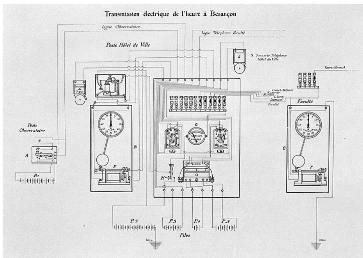
Transmission électrique de l'heure à Besançon, 1904.
