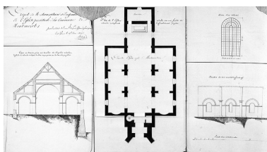
Projet de restauration et d'agrandissement de l'église paroissiale de la commune de Montmorot, vu avec la retombe du plan.
