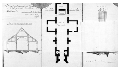
Projet de restauration et d'agrandissement de l'église paroissiale de la commune de Montmorot, vu sans la retombe du plan.
