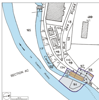
Plan-masse et de situation. Extrait du plan cadastral, 1982, section ZN, 1:2000 agrandi à 1:1000. Dess. André Céréza IVR43_20022501330NUDA
