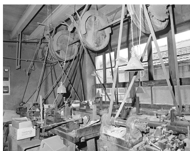
Partie de l'atelier utilisée pour la finition des pipes. Phot. Jérôme Mongreville IVR43_19963901072X
